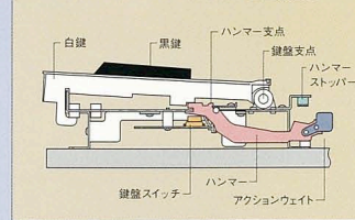
アドバンスド・ハンマー・アクション 鍵盤断面図
